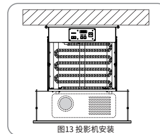
图13 投影机安装
