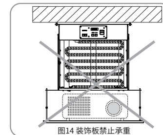
图14 装饰板禁止承重
