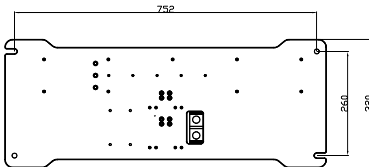
俯视图
