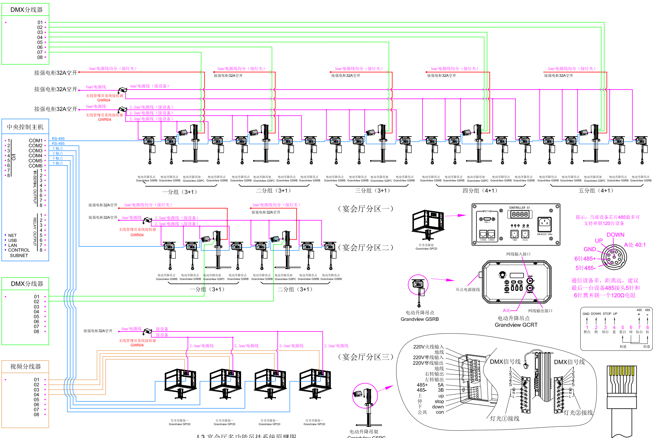
电动升降吊点、电动升降吊架接线详图
